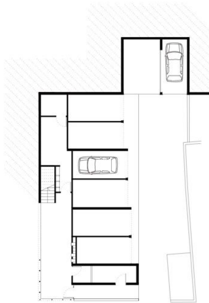
Plan RDC
